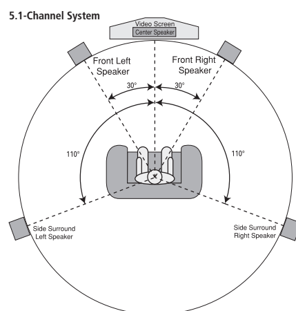
B. Avståndet mellan vänster och höger högtalare ska vara detsamma som avståndet från sittplatsen till visningsskärmen. Prova också att placera vänster och höger högtalare något framför centerhögtalaren.
